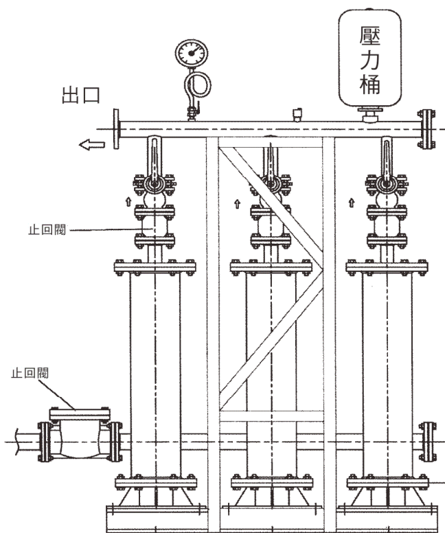
管中泵浦立式並聯安裝
